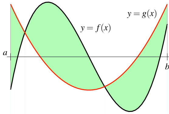
El área de la figura es \int_a^b |f(x) - g(x)| dx
