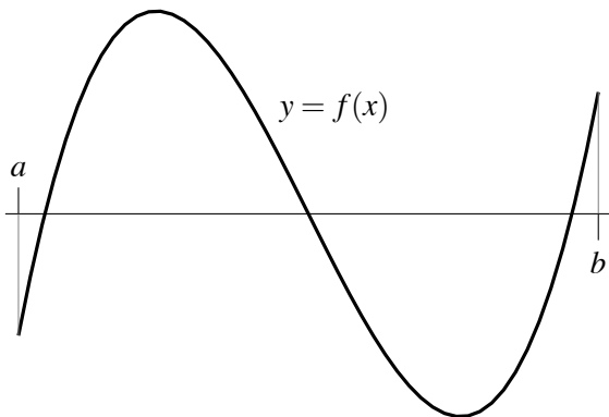
La longitud de la curva es \int_a^b \sqrt{1 + f'(x)^2} dx
