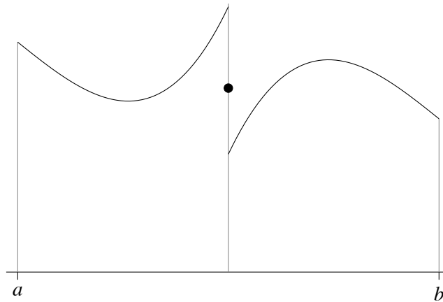
Función continua a trozos y monótona a trozos
