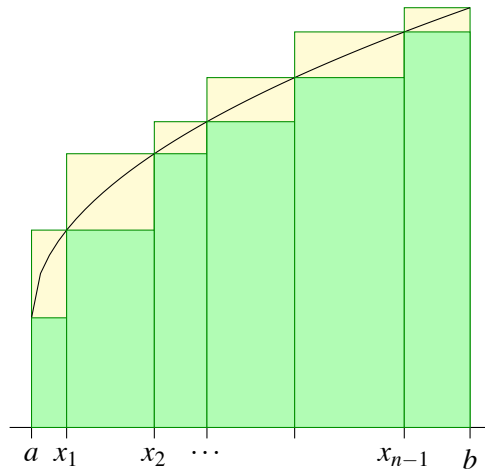
Suma superior y suma inferior para una función monótona
