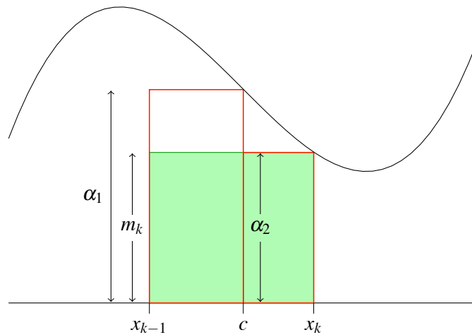
Diferencia entre las sumas inferiores correspondientes a P y Q
