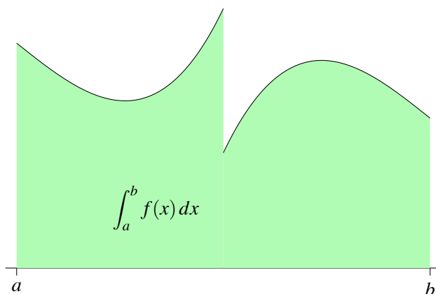
La integral y el área
