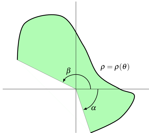
El área de la figura es \frac{1}{2} \int_{\alpha}^{\beta} \rho(\theta)^2 d\theta
