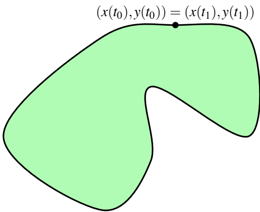
El área de la figura es \left| \int_{t_0}^{t_1} y(t)x'(t) dt \right| , si la curva es cerrada
