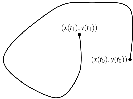
La longitud de la curva es \int_{t_0}^{t_1} \sqrt{x'(t)^2 + y'(t)^2} dt
